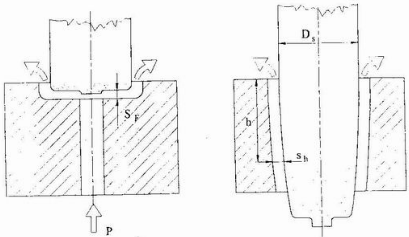
9.9. ábra. A szikraforgácsolt lyuk hossz-szelvényének alakja
