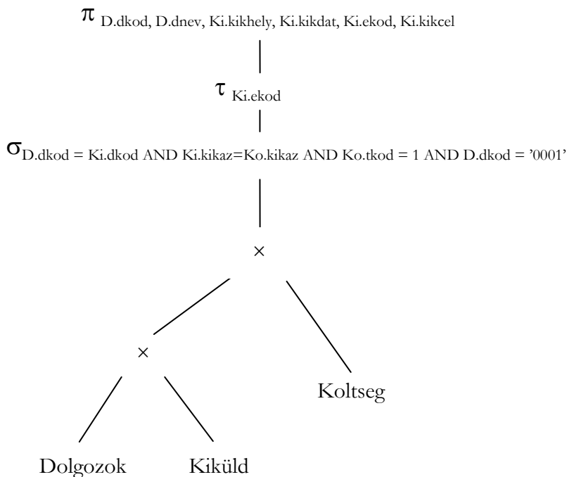
6.1. ábra. Logikai lekérdezés terve
