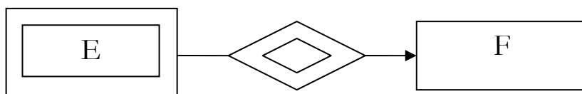
2.7. ábra. Gyenge egyedhalmaz
