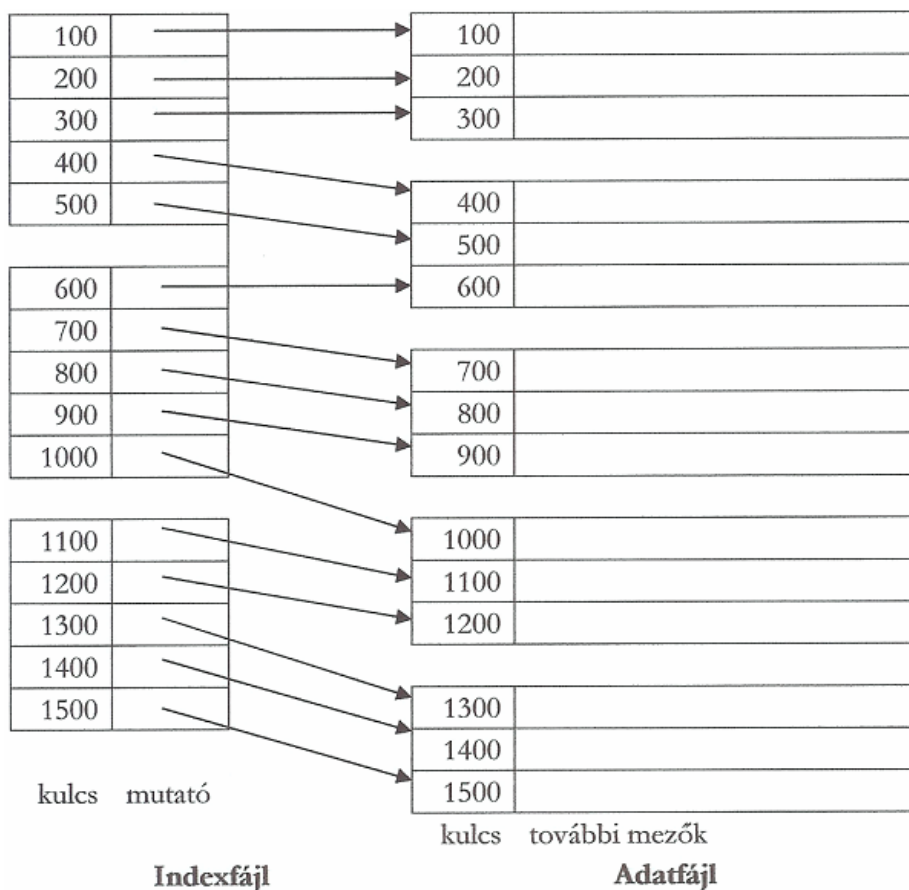
4.5. ábra. Sűrű index szekvenciális adatfájlon
